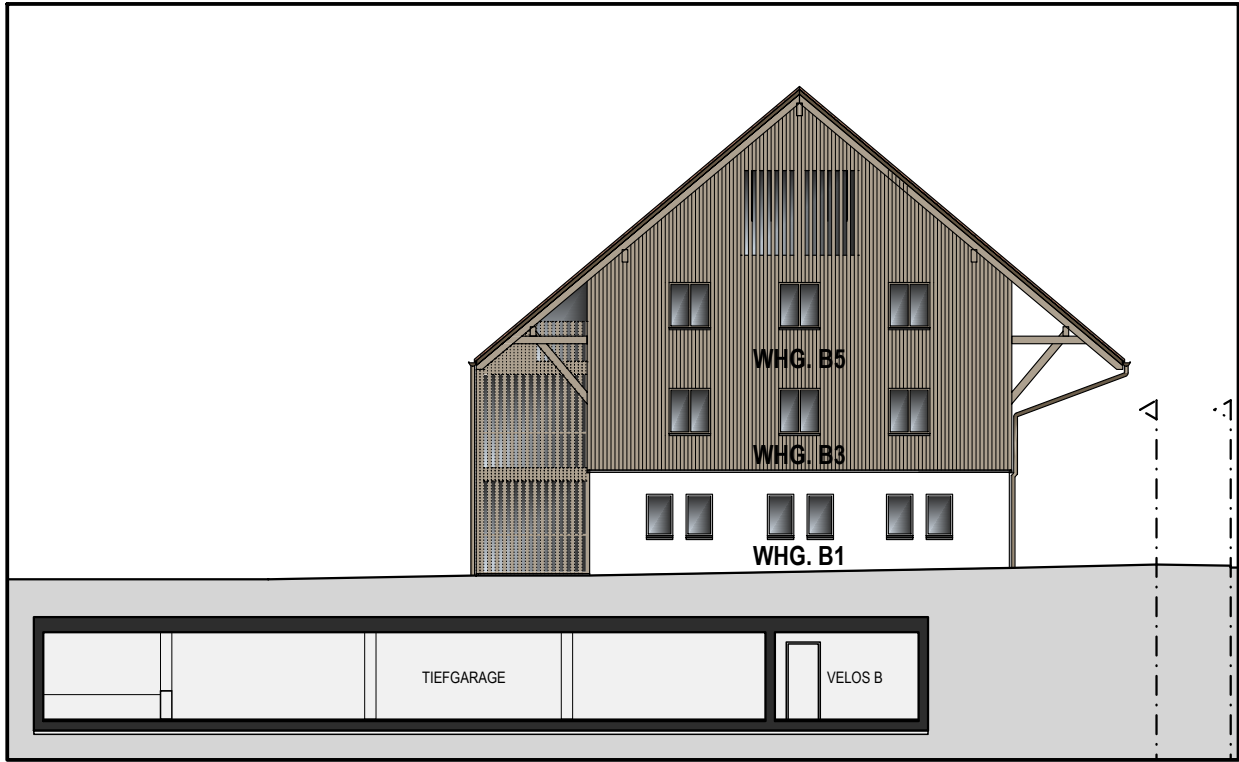
MFH B SÜD-FASSADE
